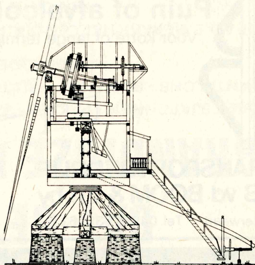
DOORSNEDE VAN EEN STANDAARDMOLEN
